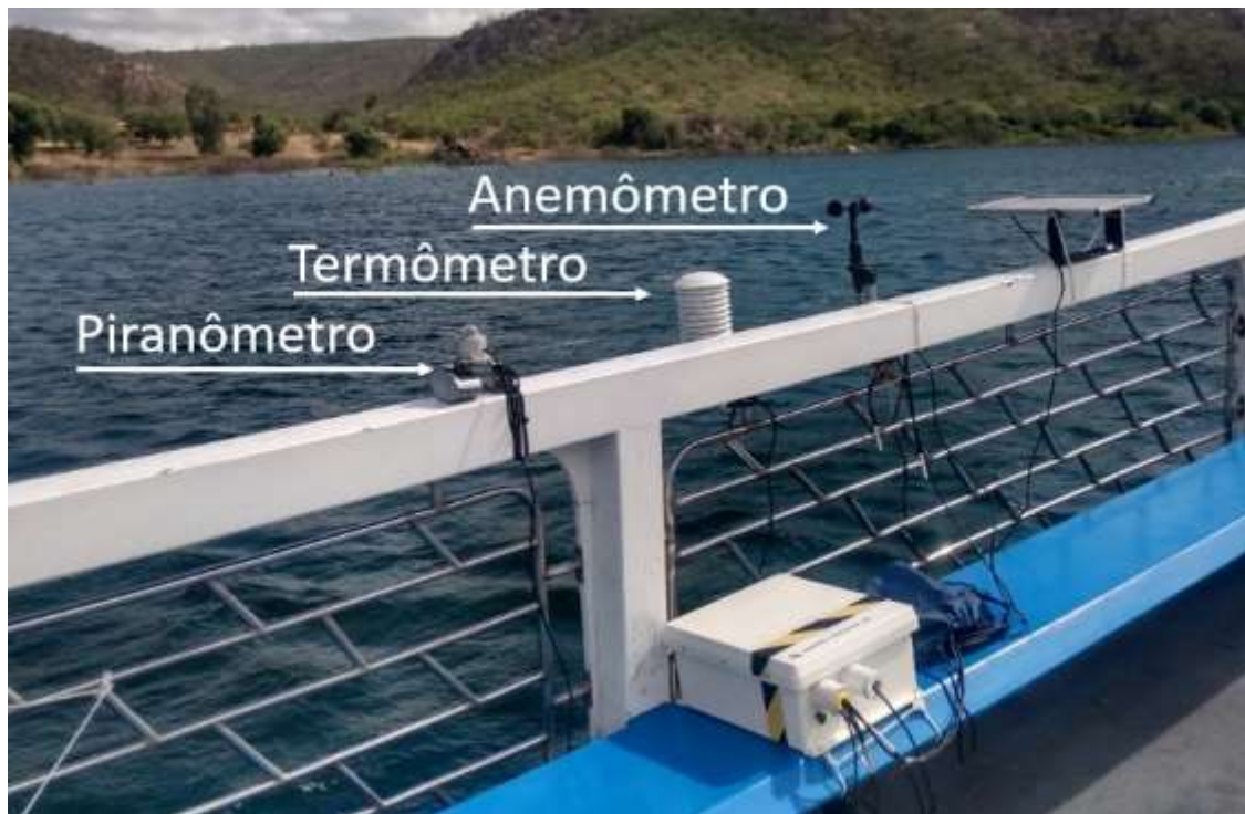
Figura 1. Sistema de observação meteorológica instalado na 3ª Expedição Científica do Baixo São Francisco.
