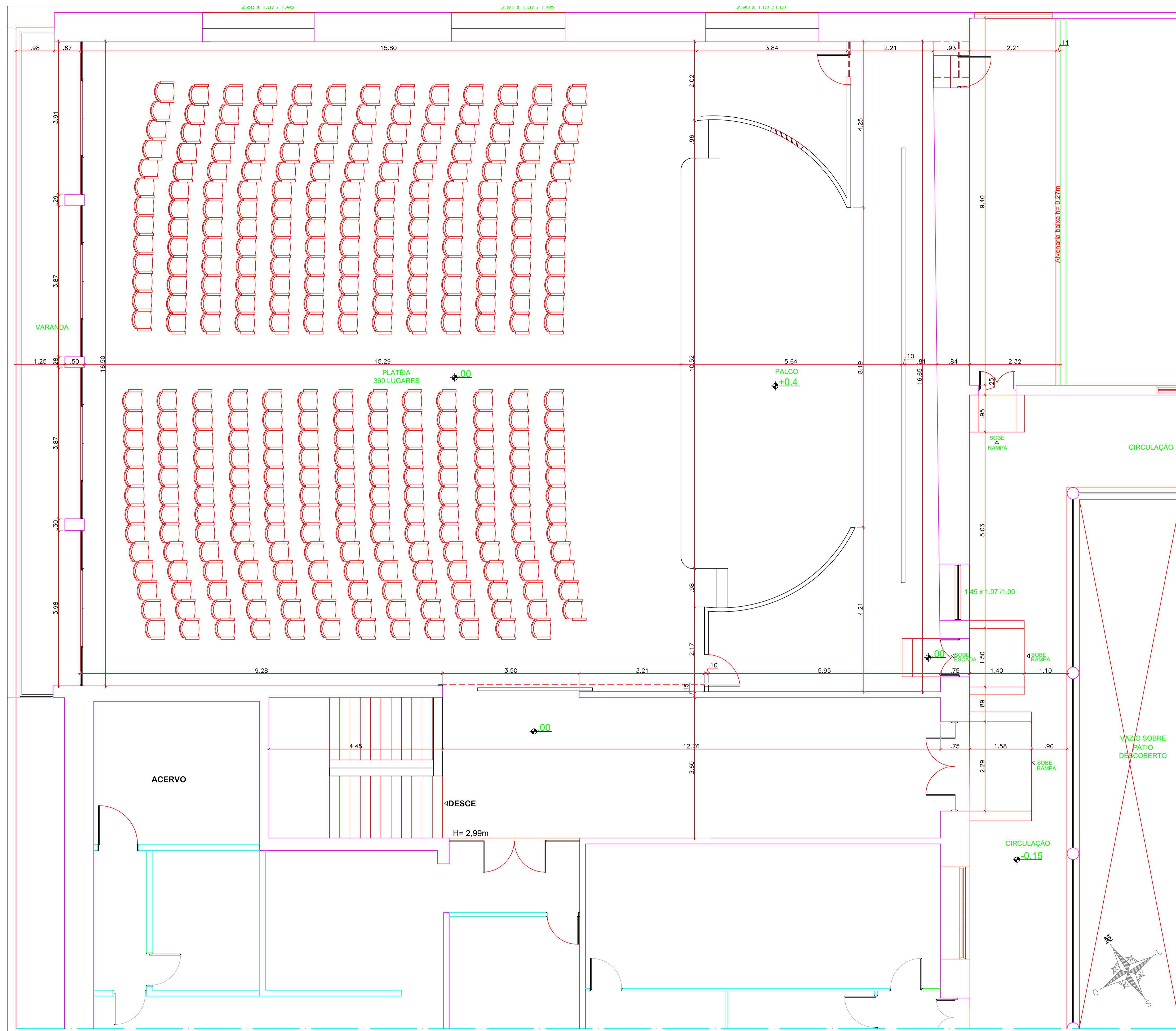
PLANTA BAIXA SITUAÇÃO ATUAL Esc: 1/50
